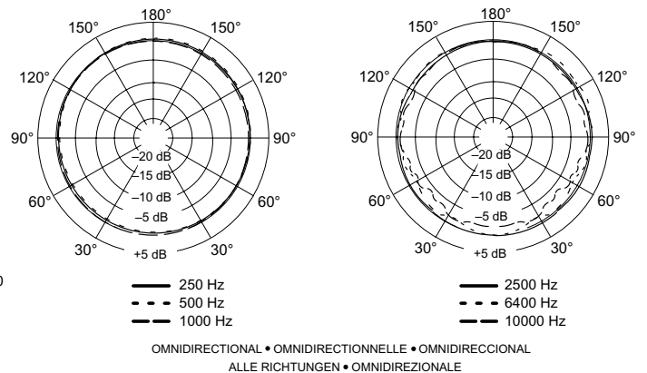
TYPICAL POLAR PATTERNS COURBES DE DIRECTIVITÉ TYPQUES TYPISCHE POLARMUSTER PATRONES DE CAPTACION POLAR TIPICOS DIAGRAMMI POLARI TIPICI FIGURE 10 • ABBILDUNG 10 • FIGURA 10
